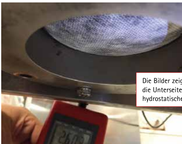
Hydrostatischer Drucktest einer SOLITEX MENTO 3000 nach fünf Jahren natürlicher Alterung unter Deckung – trocken bei 2.600 mm.
