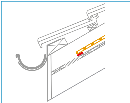
Raccord du pied de versant en cas de sollicitations normales et élevées.
